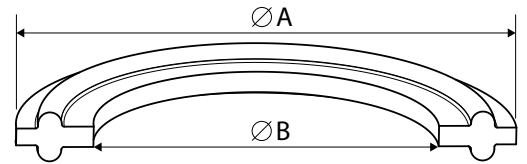
Ausführung ohne Fassungslippe (ungeflanscht) für Größen mit AD >3/4"
