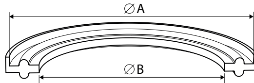
Geflanschte Dichtungen (mit Fassungslippe)
