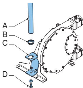
Standardní čerpadlo
