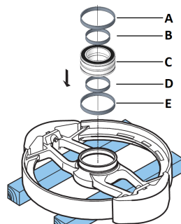
Sada ložisek pro vysokou zátěž
