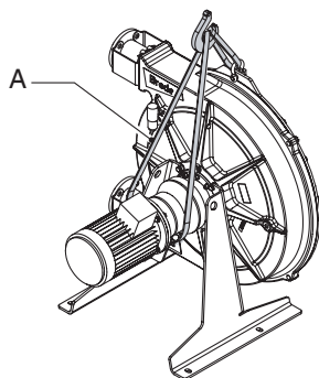
Standardní čerpadlo
