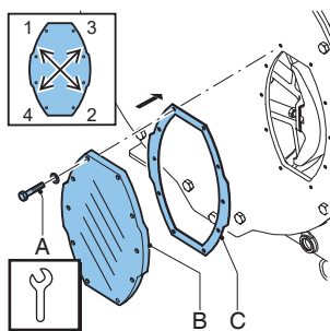
Standardní čerpadlo
