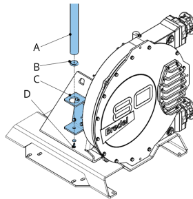
Højtydende pumpe
